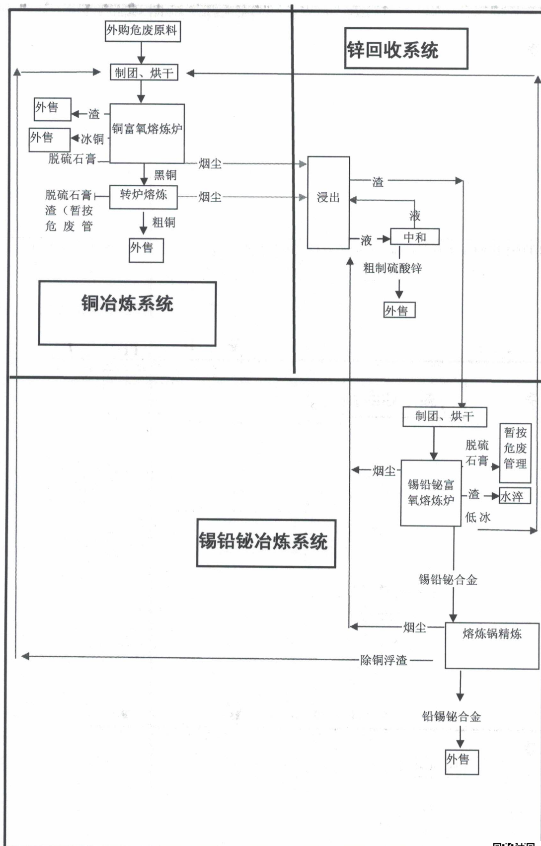
图 3-2 目前全厂工艺流程图
