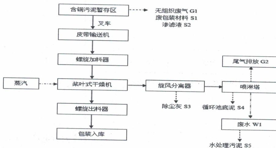
图 2 主体工程生产工艺流程图
